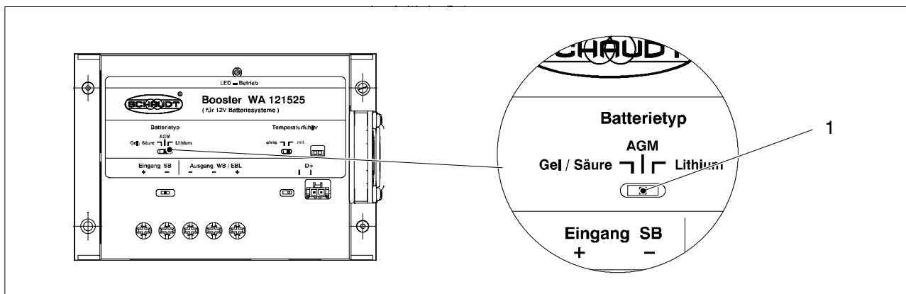
Bild 5 Batterie-Wahlschalter
